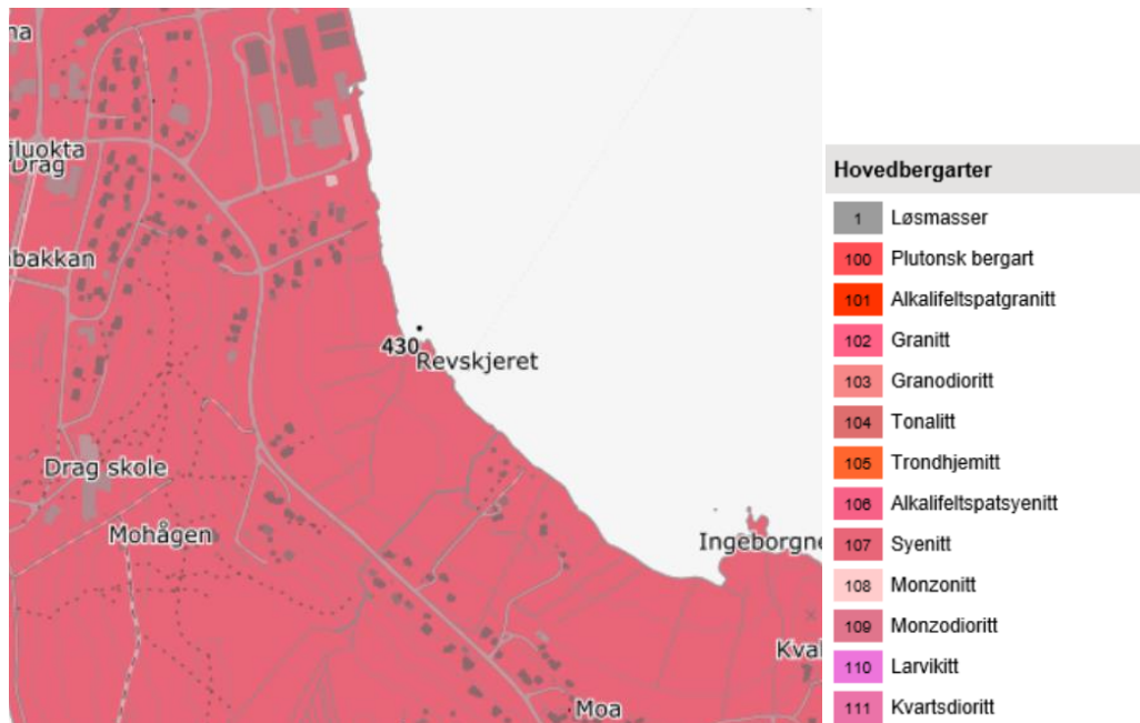
Figur 6: Bergrunnskart (5)
