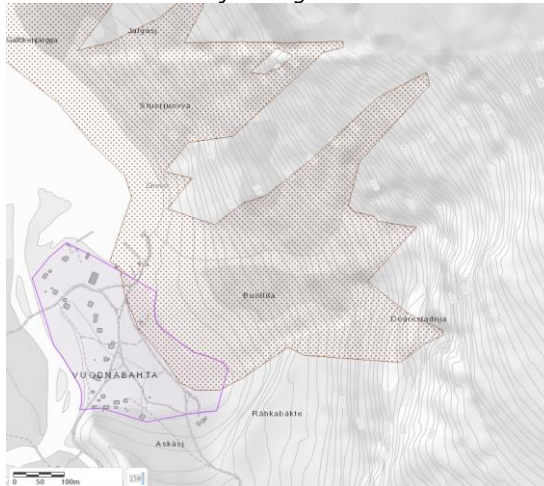
Figur 20: Aktsomhetskart. Vurdert område (lilla) ligger innenfor aktsomhetsområder for steinsprang, snøskred og jord- og flomskred.
