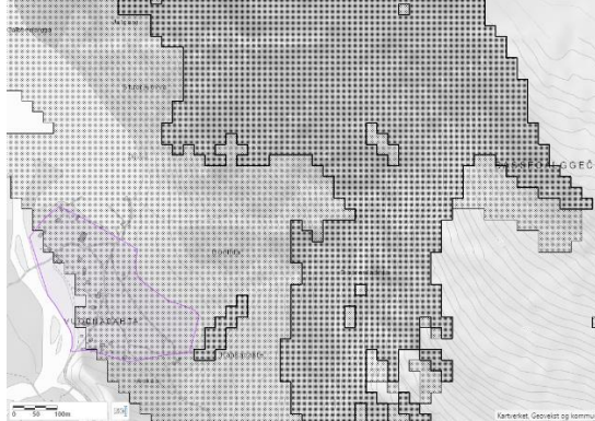
Aktsomhetsområde jord- og flomskred:
