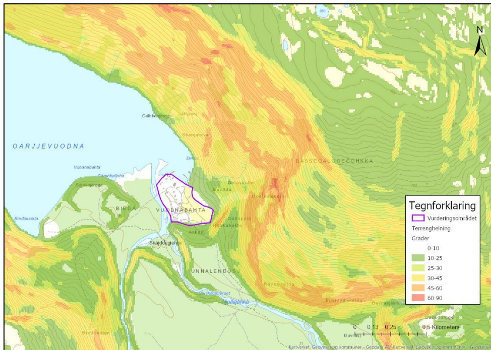
Figur 5: Helningskart generert fra terrengmodell med oppløsning 10x10 m.
